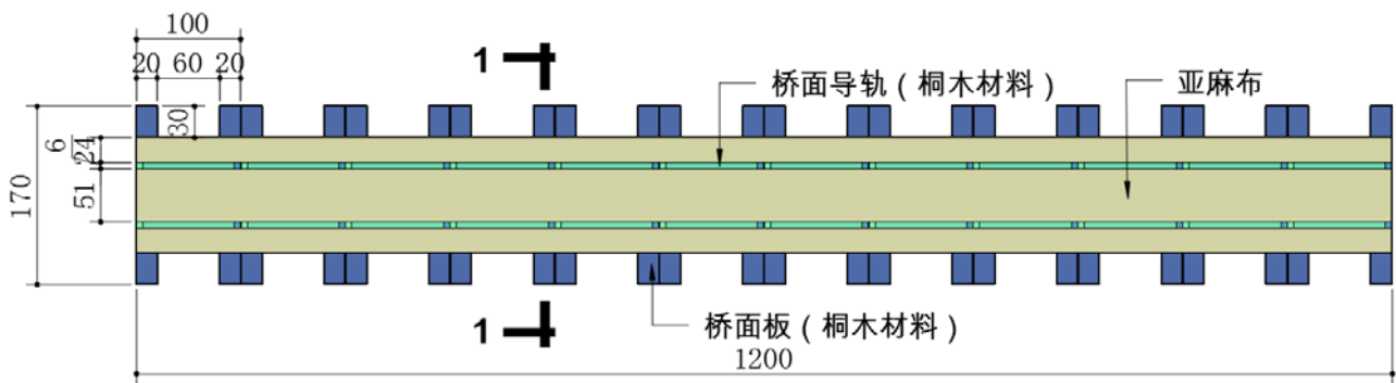
(a) 桥面板俯视图
