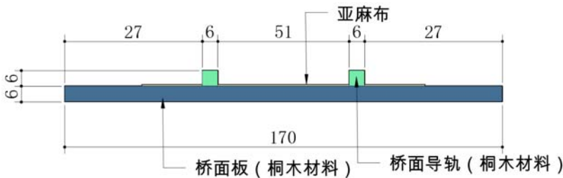
(d) 1-1 剖面图
