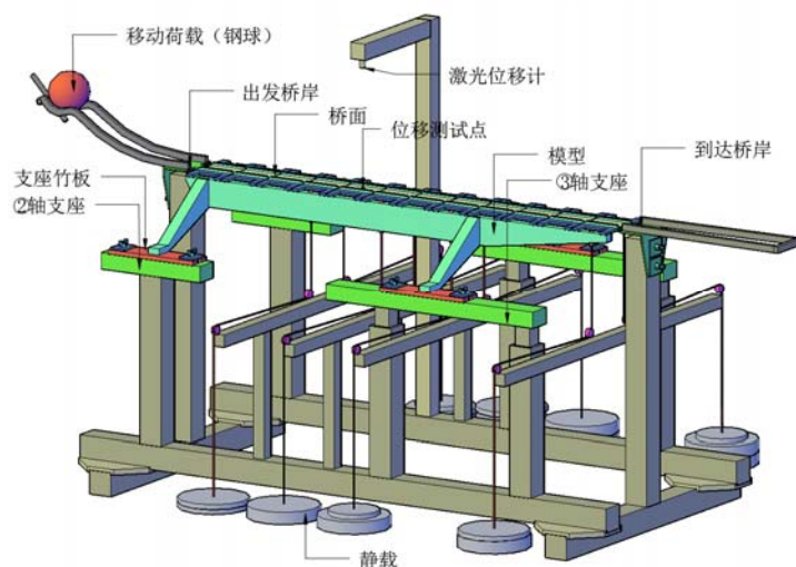
图 1 模型轴测示意图
