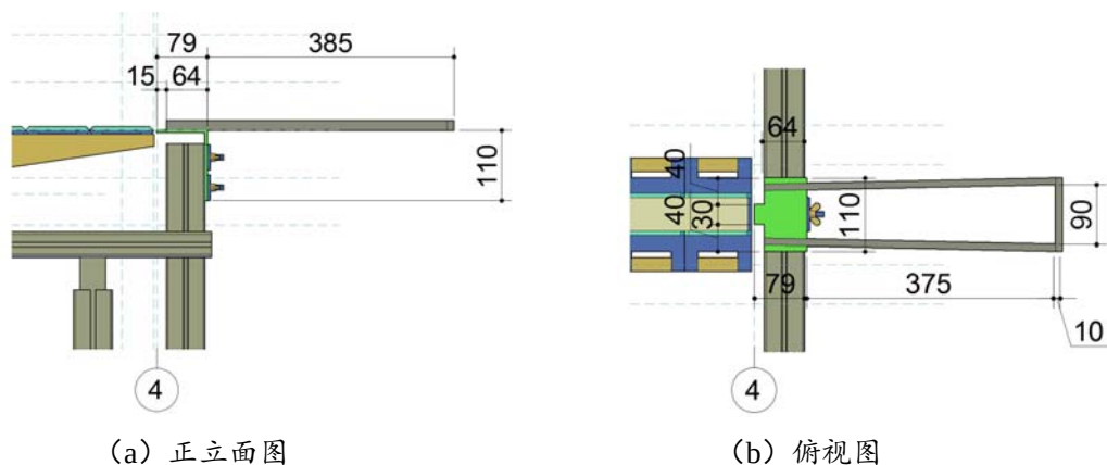
图4 到达桥岸详图
