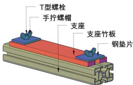
(a) 支座竹板与支座的连接方式
