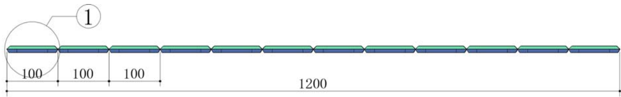
(b) 桥面板正视图
