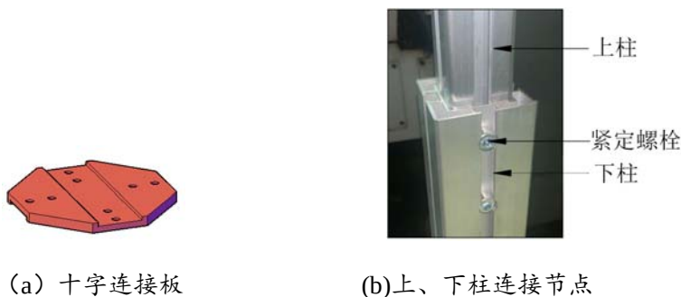
图10 特殊节点示意图
