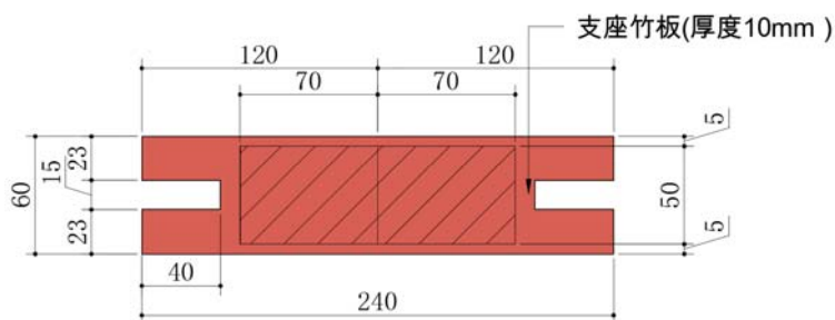
(b) 支座竹板详图
